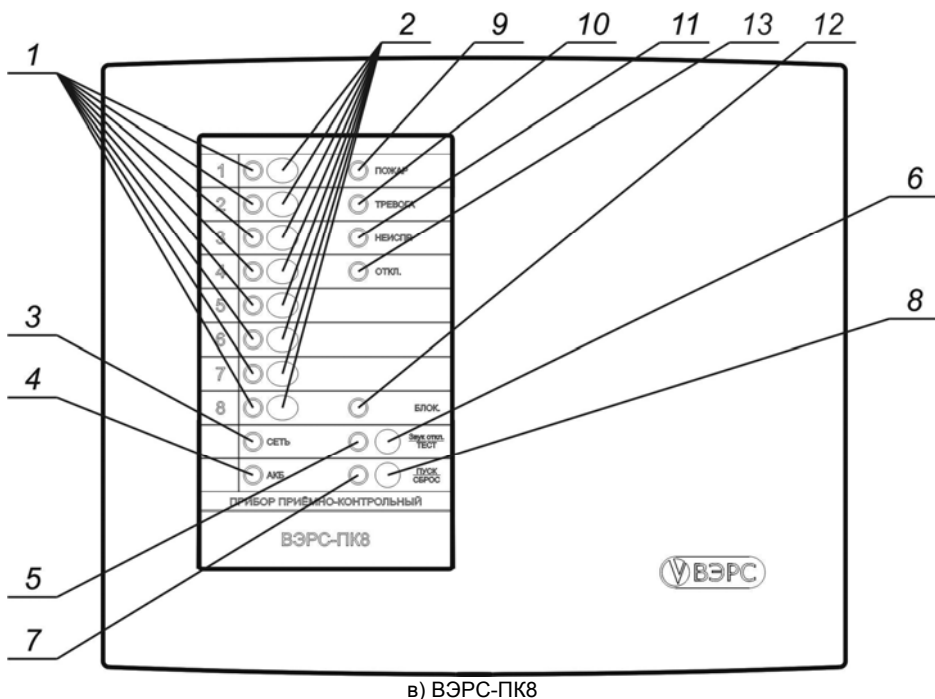
Рисунок А1. Внешний вид передней панели приборов ВЭРС-ПК(8,4,2) П(Т)(LAN)(-РС) Версия 3.2.)
