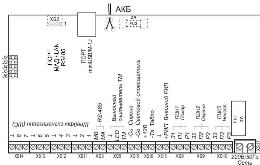
Рисунок Б2. Вид на клеммы и разъемы для внешних подключений ВЭРС-ПК(8,4,2)(П,М)(Т)(LAN)(-РС) Версия 3.2.
