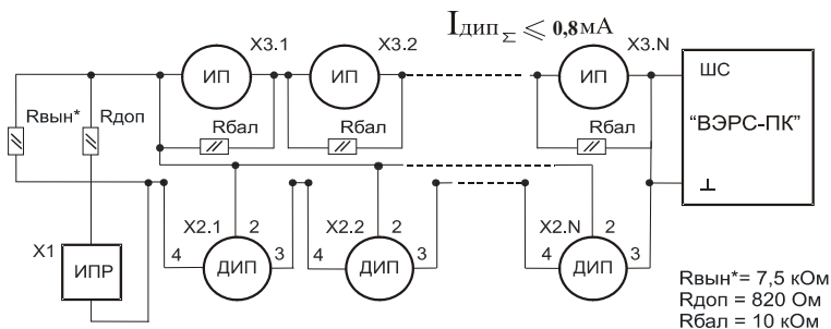
Рисунок.Б8. Комбинированная схема включения ШС. Однопороговый алгоритм с верификацией.
