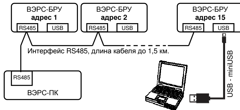
Рисунок А6. Структурная схема связи приборов ВЭРС-БРУ с ВЭРС-ПК(2,4,8,16,24) Версия 3.1.
