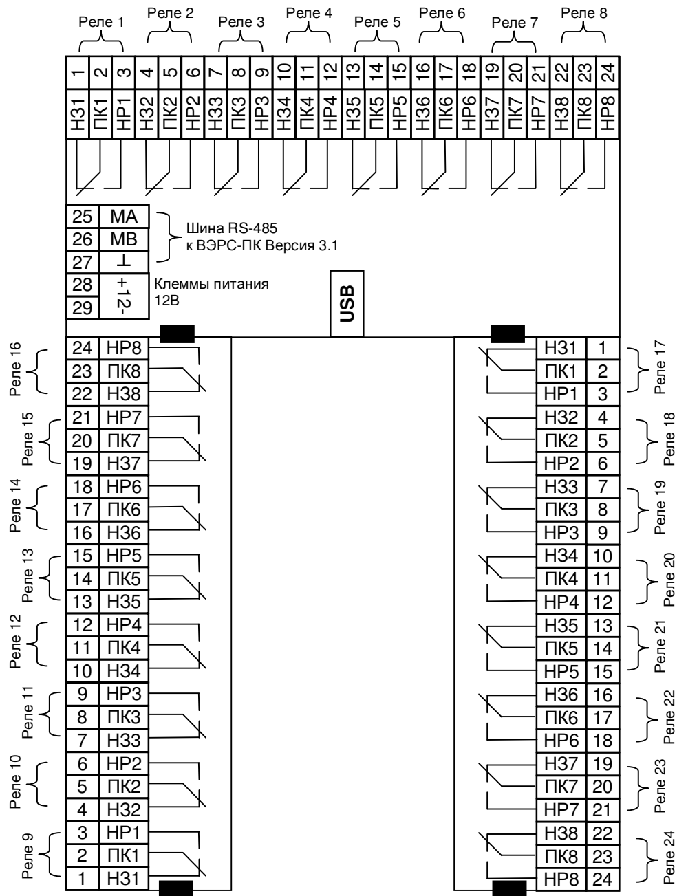
Рисунок А5. Схема внешних соединений ВЭРС-БРУ.
