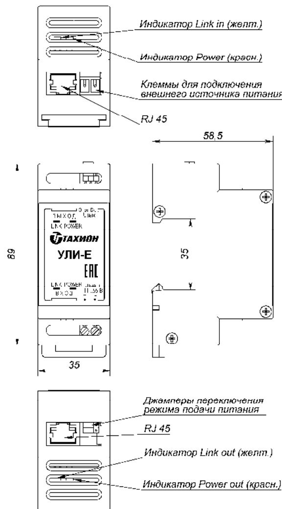
Рис.2 Внешний вид и габаритные размеры.
