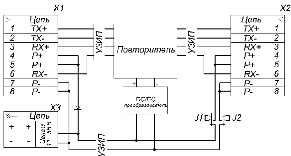
Рис.1 Структурная схема УЛИ-Е.
