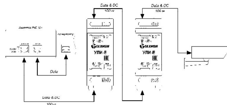
Рис.6 Пример удлинения линии связи с использованием комплекта питания PoE-12 или аналогичного.
