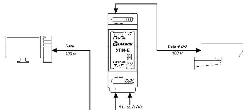
Рис.4 Подключение IP видекамеры через УЛИ-Е.
