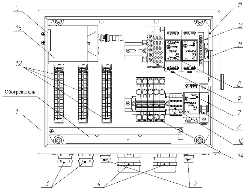
Рис. 1. Устройство термошкафа (дверь открыта на 90°)
