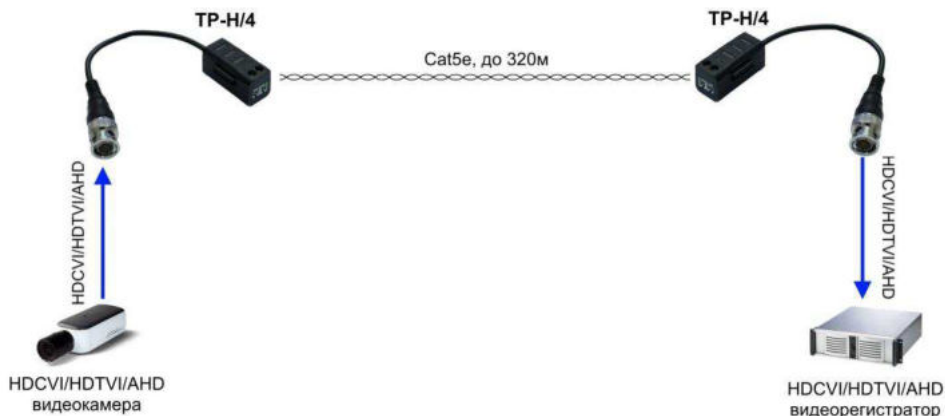
Рис.5 Схема подключения приемопередатчиков TP-H/4
