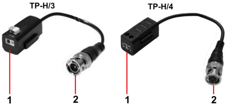
Рис. 3 Приемопередатчики TP-H/3, TP-H/4, разъемы
