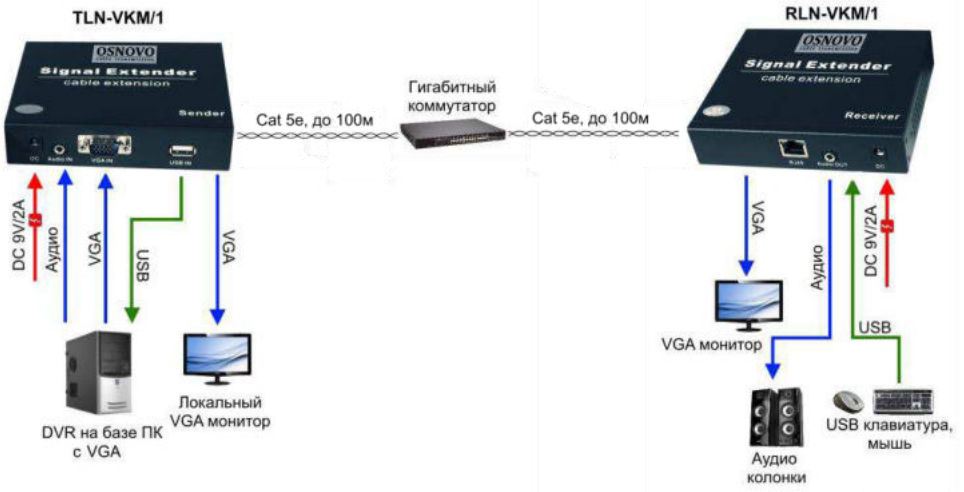
Рис. 5 Схема подключения комплекта TLN-VKM/1+RLN-VKM/1 в режиме «точка-точка» через гигабитный коммутатор
