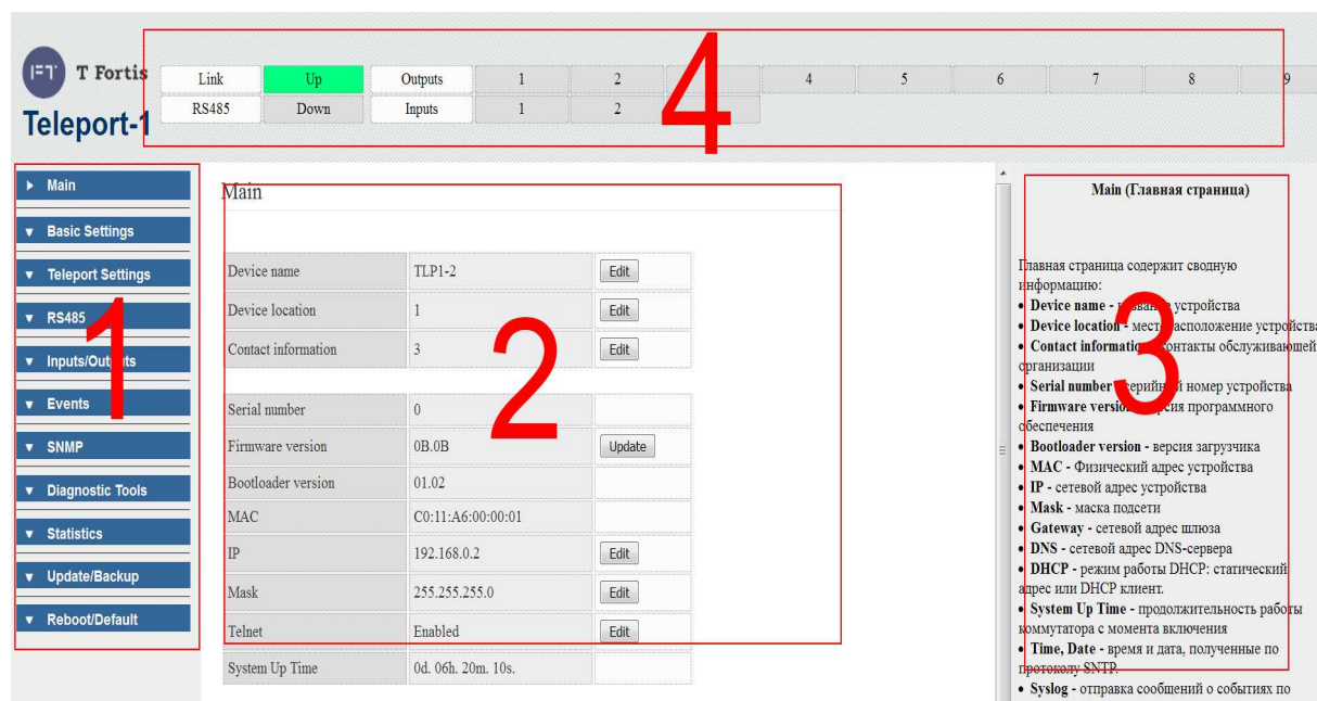
Рис. 5.3.1.2. Web-интерфейс
