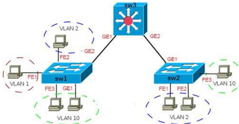
Рис. 5.3.14.1 Топология сети
