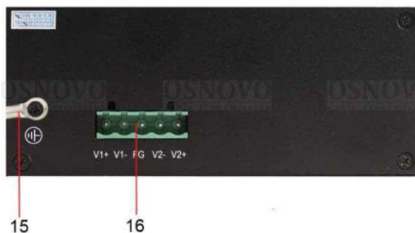
Рис. 3 Разъемы и индикаторы коммутатора SW-8082/IC
