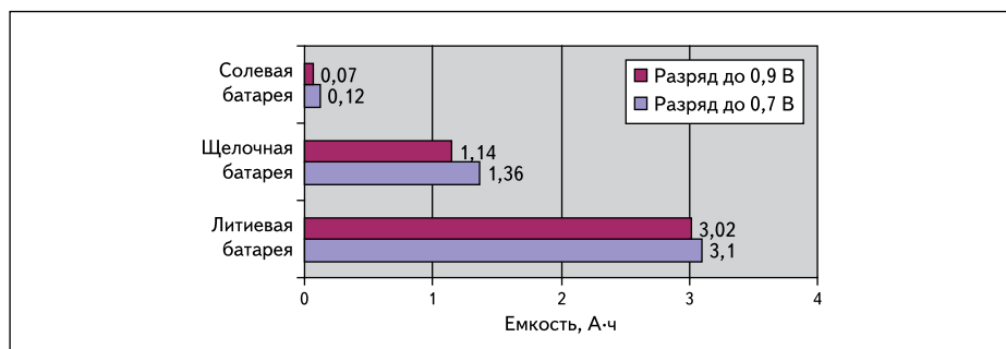
Рис. 1. Диаграмма разряда с постоянным током 750 мА
