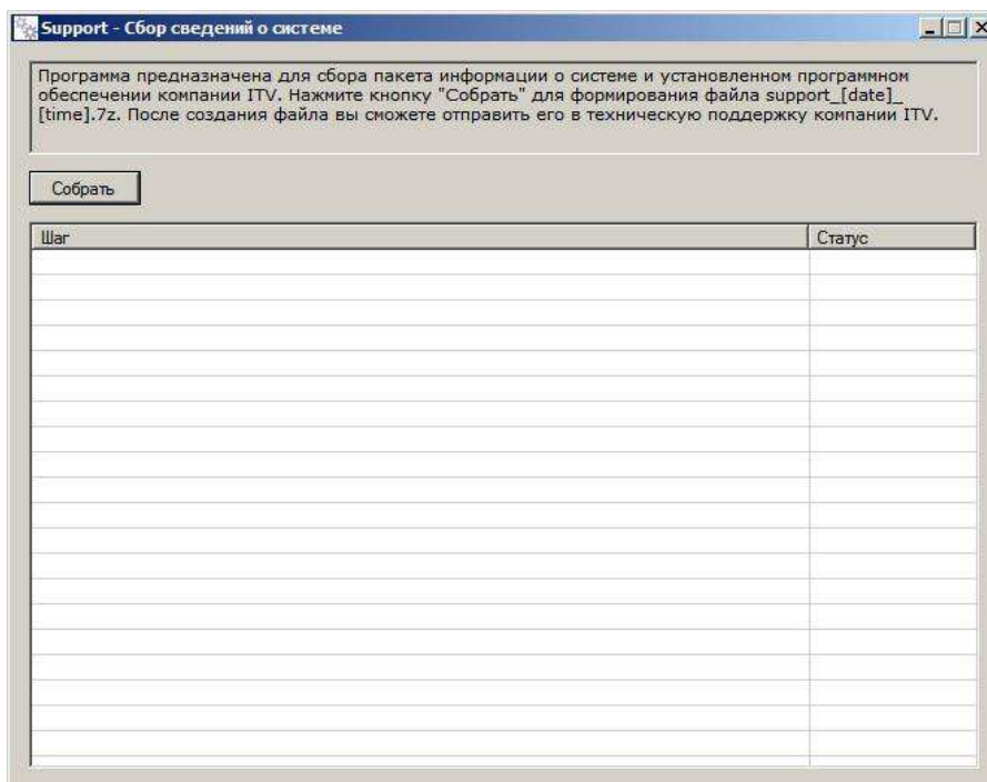
Рис. 7 Утилита Support
