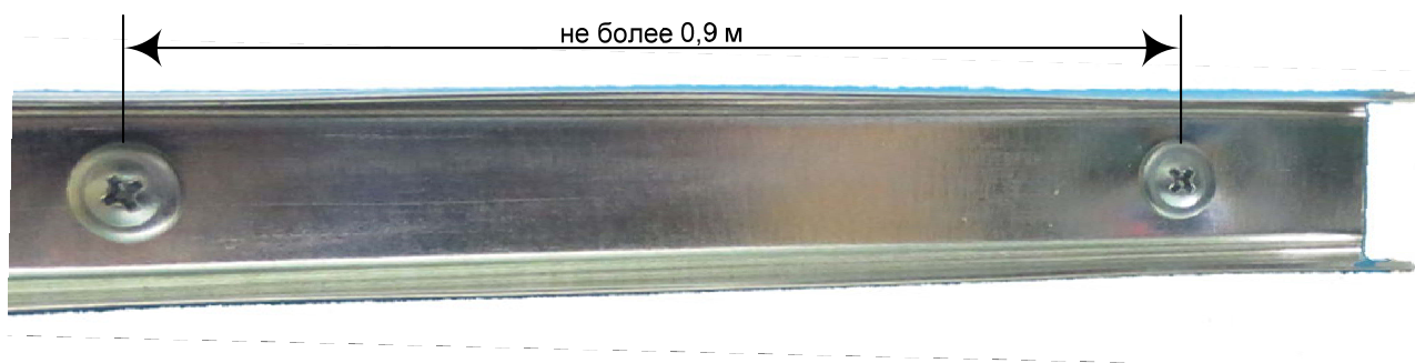
Рис. 16. Крепление короба.
