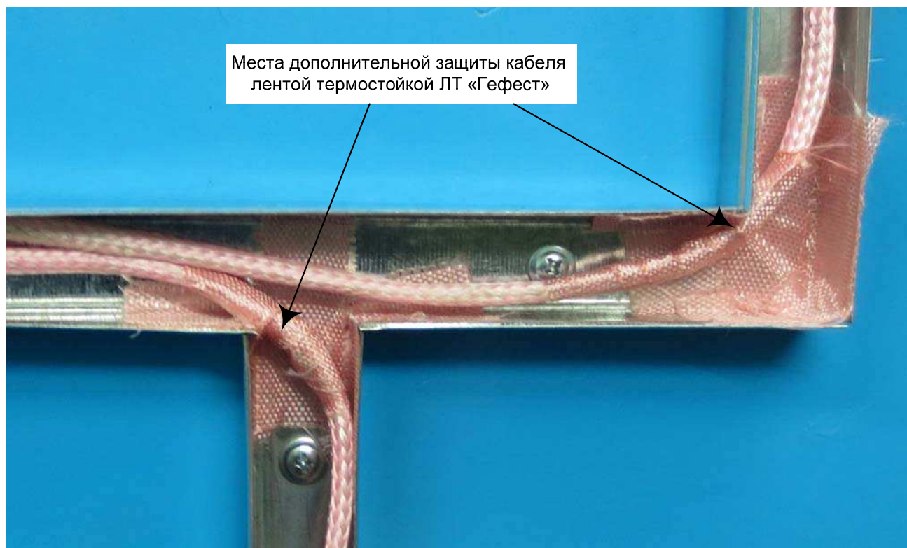
Рис. 18. Укладка КГО «Саламандра» в КМО.
