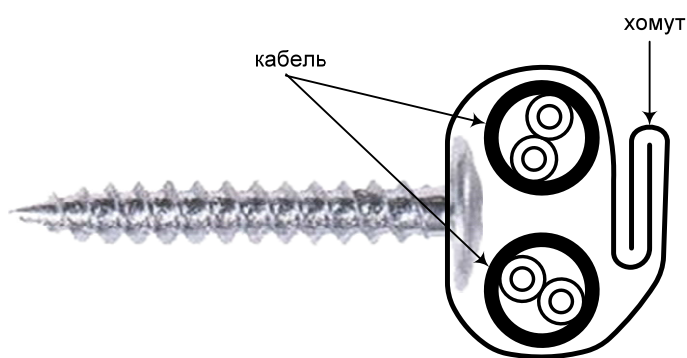
Рис. 7. Установка дюбель-хомута КФСТ.735322.041. Вариант 3.
