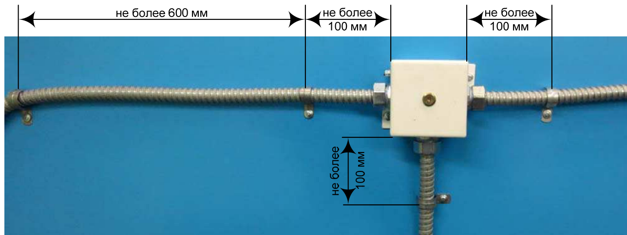
Рис. 15. Прокладка КЛ в металлическом рукаве.
