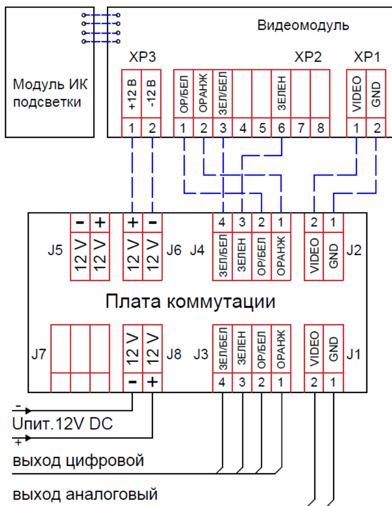
Рисунок 4 – Схема подключения камеры с питанием 12 В (исполнение без PoE)
