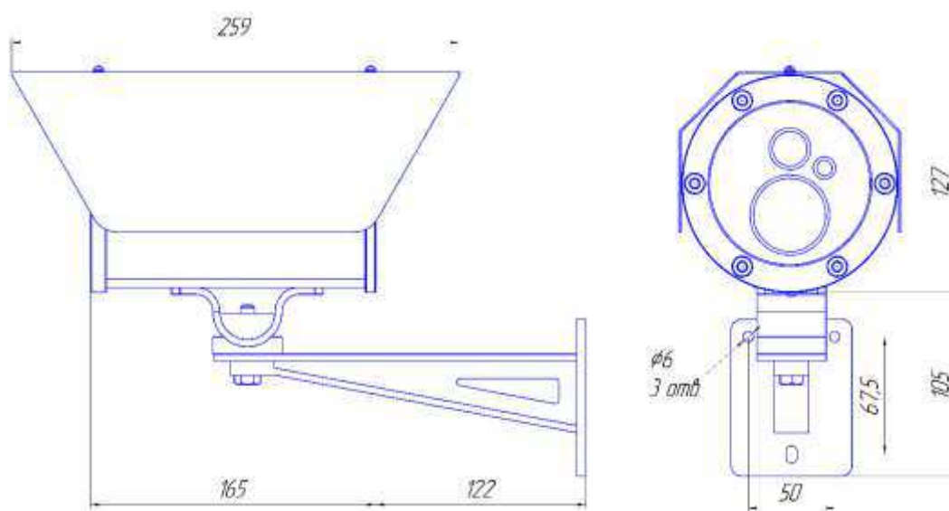
Рисунок 1 – Габаритные размеры видеокамеры
