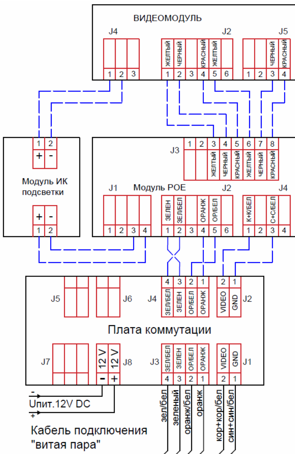
Рисунок 3 – Схема подключения камеры с питанием по PoE или 12V
