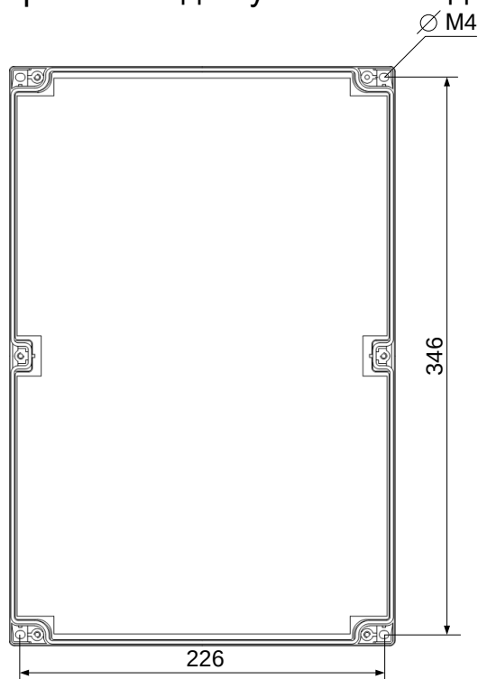
Рис. 6.1. Разметка крепления
