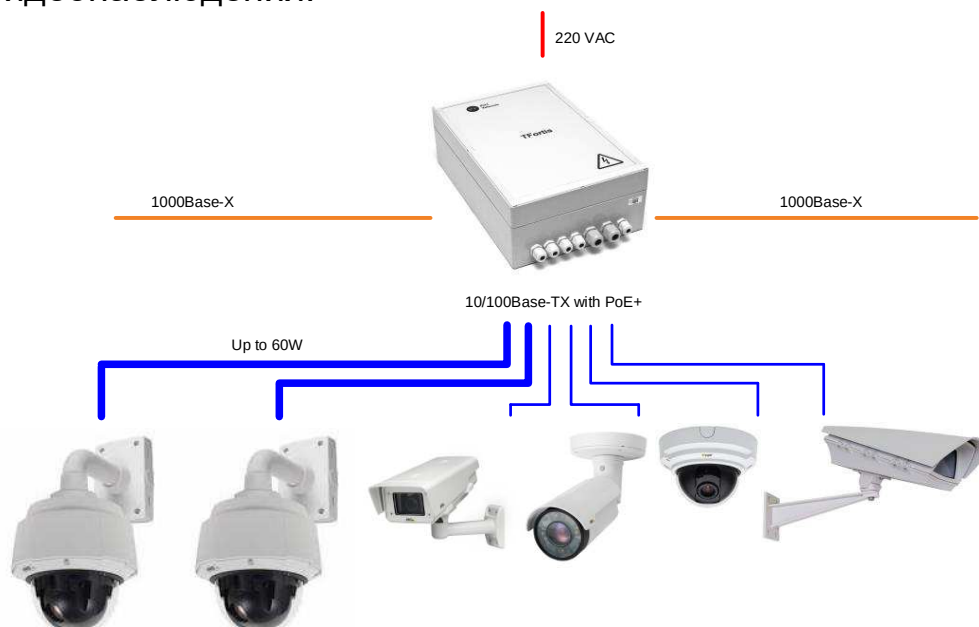
Рис. 1. Схема подключения PSW-2G6F+
