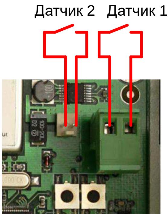
Рис. 2.6. Сухие контакты
