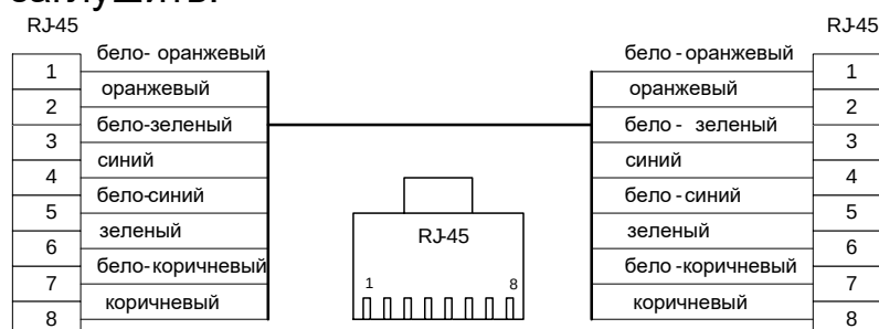
Рис. 6.4. Разделка кабеля.
