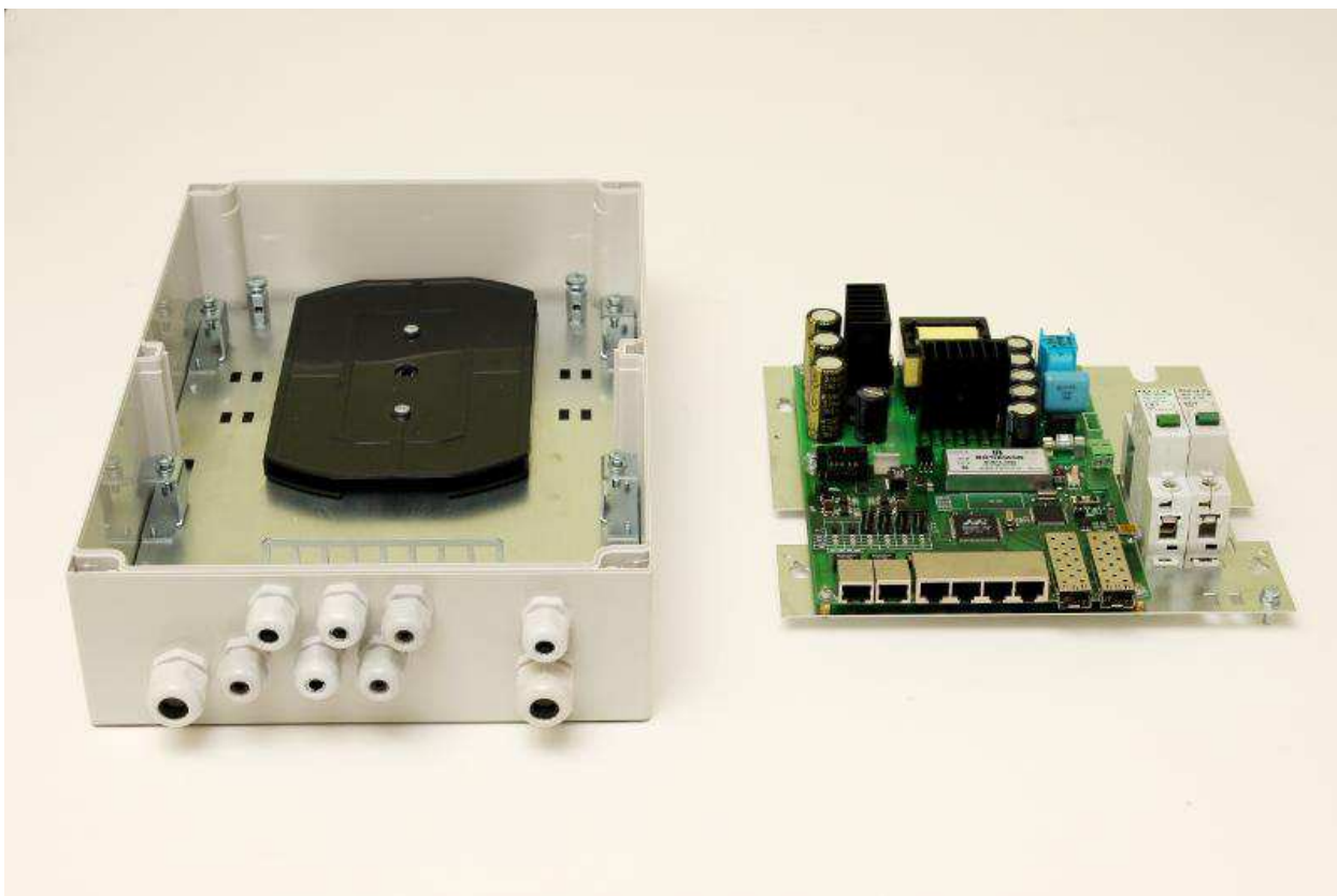
Рис. 2.1-3. PSW-2G+ - в разборе
