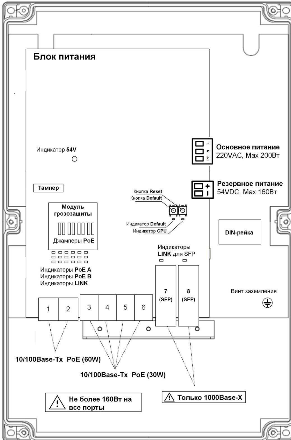
Рис. 2.2. Расположение элементов PSW -2G6F+
