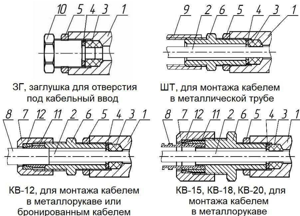
Рисунок 12 – Вводные устройства с одинарным уплотнением
