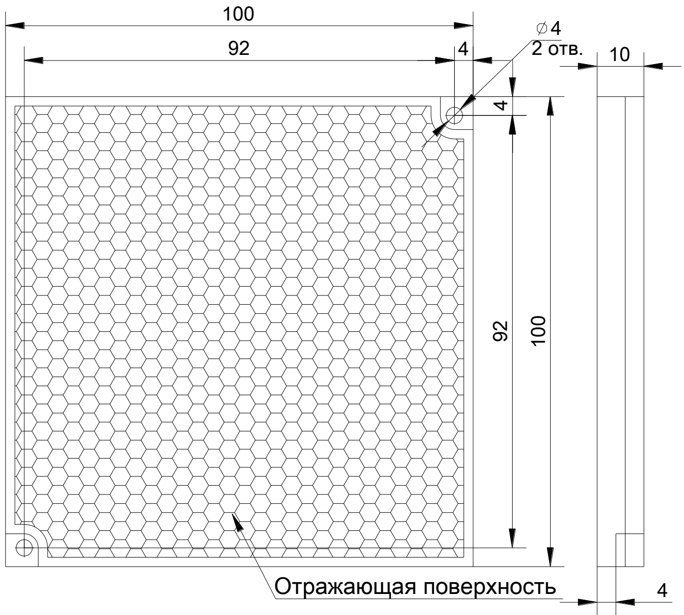
Рисунок 1 Общий вид отражателя
