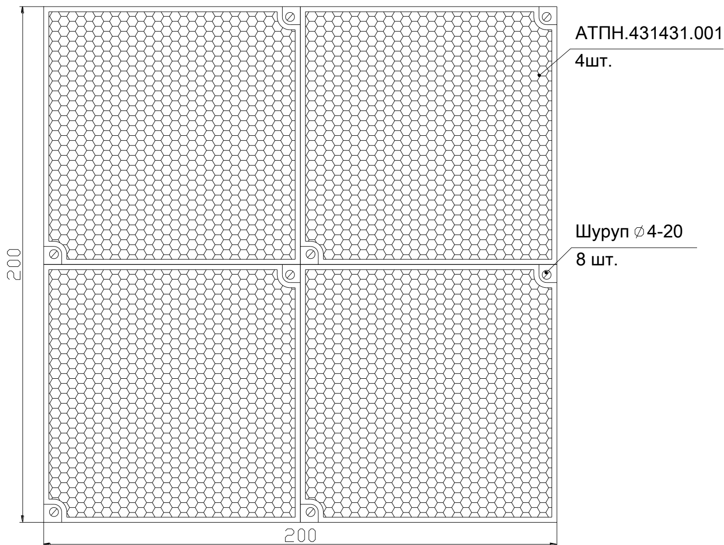
Рисунок 2 Монтажный чертеж четырех отражателей
