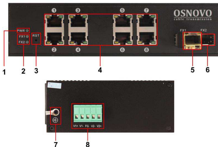
Рис. 4 Промышленный коммутатор SW-8091/IC, разъемы, кнопки и индикаторы
