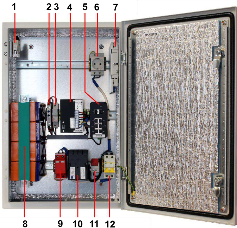
Рис.2 Уличный коммутатор с системой обогрева и резервным питанием, внутренние компоненты, на примере модели OS-46TB1(SW-60602/ILC)
