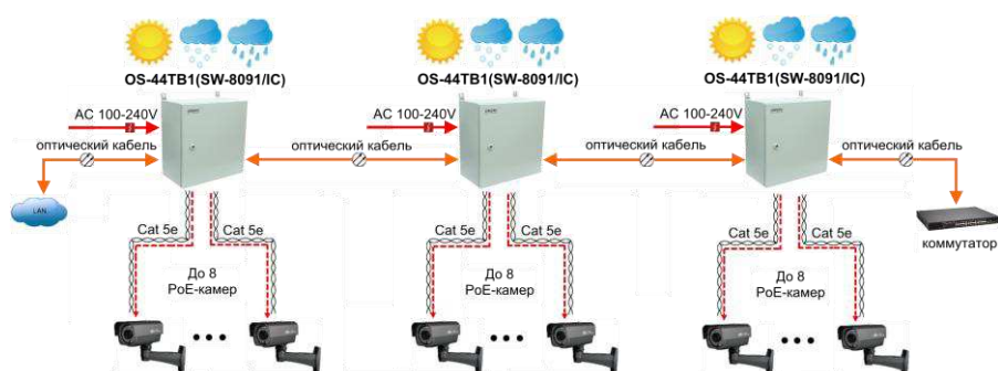
Рис. 3 Типовая схема подключения уличных коммутаторов на примере модели OS-44TB1(SW-8091/IC)
