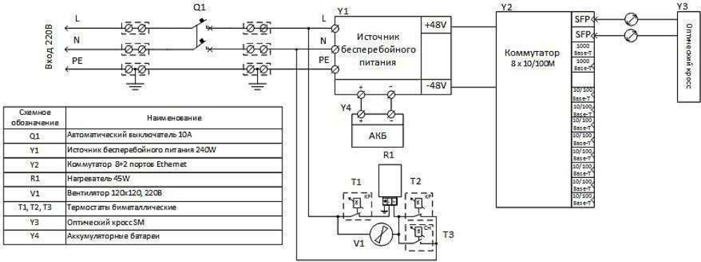
Рис. 1.Электрическая схема Узла доступа NSBox-280-R
