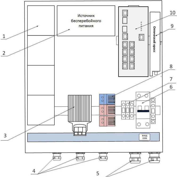
Рис. 2. Базовая комплектация Узла доступа NSBox-280-R*
