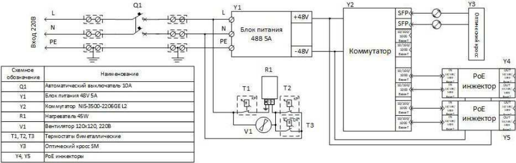
Рис. 1.Электрическая схема Узла доступа NSBox-264
