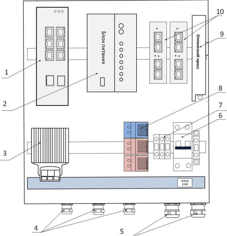
Рис. 2. Базовая комплектация Узла доступа NSBox-264*
