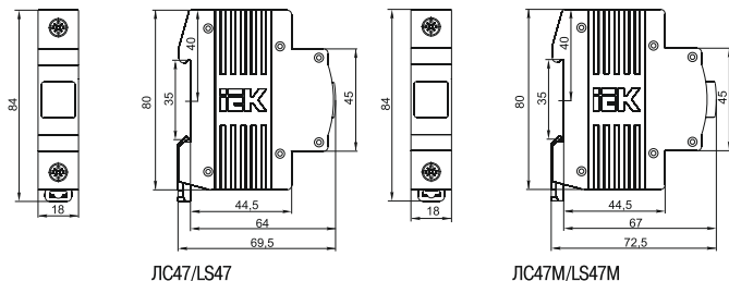
Рисунок 1 Габаритные размеры / figure 1 Overall dimensions.
