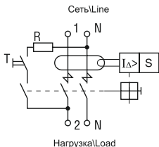
Рисунок 1. Схема электрическая принципиальная двухполюсных выключателей/ Figure 1. Electric schematic diagram of 2-pole circuit breakers
