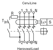
Рисунок 2. Схема электрическая принципиальная четырехполюсных выключателей/ Figure 2. Electric schematic diagram of 4-pole circuit breakers
