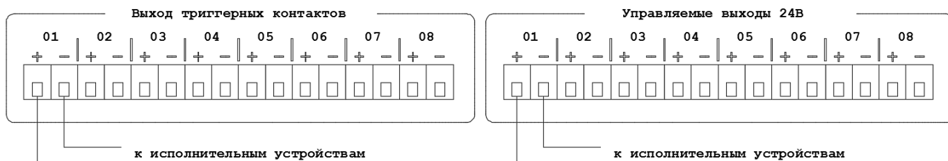
Рис. 3.6. Схема подключения внешних исполнительных устройств к LPA-DUO.
