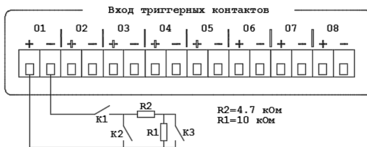
Рис. 3.4. Схема подключения внешних сигналов управления к LPA-DUO с контролем целостности
