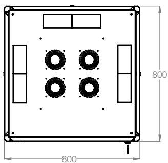
ВИД СВЕРХУ
