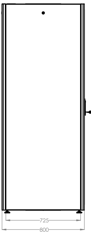
ВИД СБОКУ
