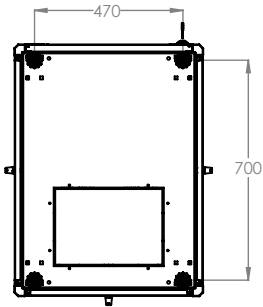
ВИД СНИЗУ
