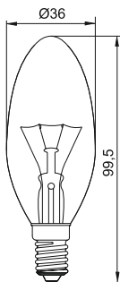
Рисунок 2. Лампа С35 цоколь E14
