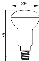
Рисунок 16 – Лампа LED-R50, 5 Вт, цоколь E14
