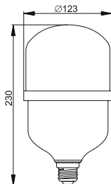
Рисунок 22 – Лампа LED-HP, 50 Вт, цоколь E27
