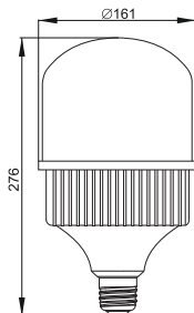
Рисунок 24 – Лампа LED-HP, 65 Вт, цоколь E40
