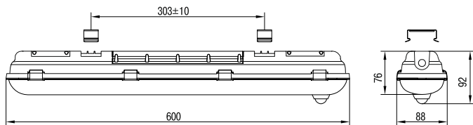
Рисунок 2. Габаритные размеры светильника ДСП 1302Д
