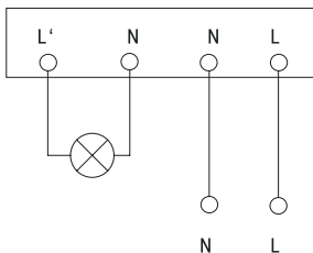
Рисунок 16 – Схема подключения датчика ДД-026
