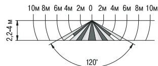
Рисунок 1 – ДД-025, ДД-201, ДД-301
