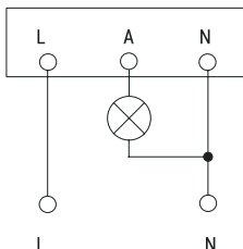
Рисунок 18 – Схема подключения датчика ДД-301
