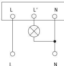
Рисунок 19 – Схема подключения датчика ДД-401
