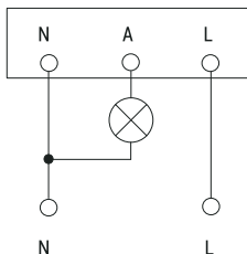
Рисунок 15 – Схема подключения датчика ДД-025, ДД-027
