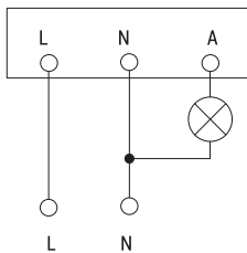
Рисунок 17 – Схема подключения датчика ДД-201
