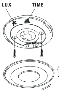
Рисунок 12 – Датчик движения ДД-026
