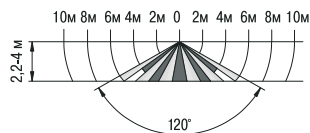
Рисунок 1 – ДД-025, ДД-201, ДД-301
