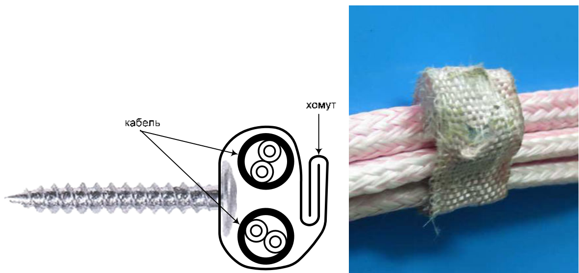
Рис. 7. Установка дюбель-хомута КФСТ.735322.041. Вариант 3.
