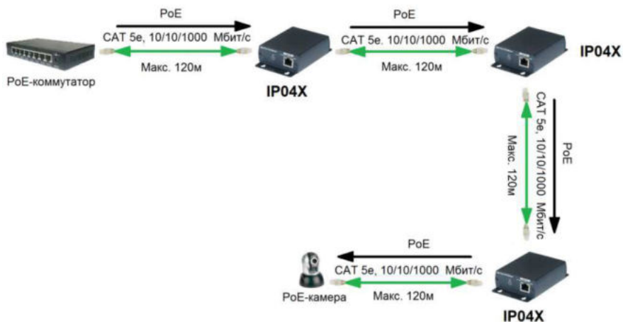
Рис.6 Схема подключения IP04X (IP04X-SO подключается аналогично)
