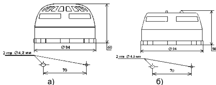
Рисунок 1. Габаритные и установочные размеры извещателей:
