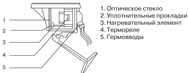
Схема установки
