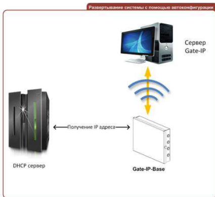
Рис.5. Автоконфигурация устройства
