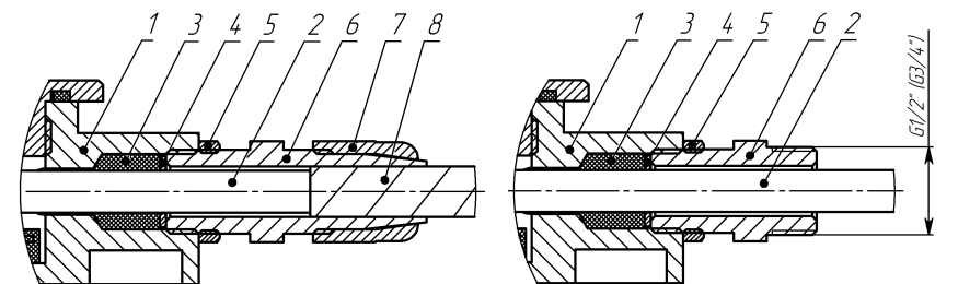
а) монтаж бронированным кабелем в кабельном вводе КВБ12
