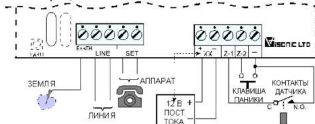
Рисунок 5. Электрические соединения DL-125C.
