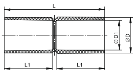
Рисунок 5 – Муфта труба-труба
