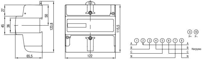
Рисунок 1 – Габаритные и присоединительные размеры счётчиков габарита 2
