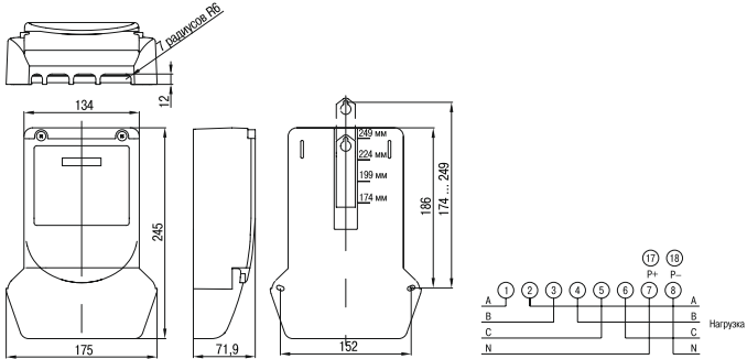
Рисунок 4 – Схема прямого подключения счётчиков габарита 4
