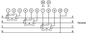
Рисунок 6 – Схема трансформаторного подключения счётчиков габарита 2.2 и 4
