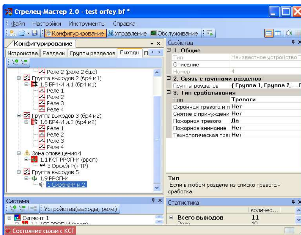
Рисунок 16 Настройка "Сирены-Р" для срабатывания по условиям сегмента ИСБ
