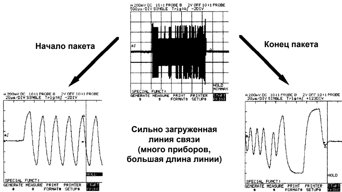
Рисунок 34 Типичная осциллограмма сигнала при большой нагрузке линии связи
