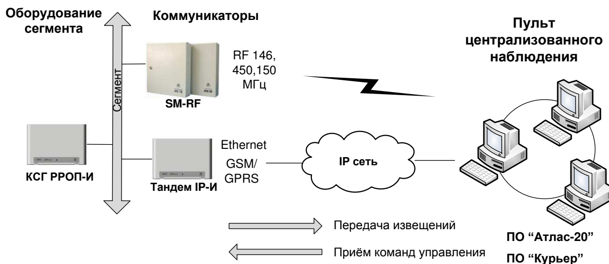
Рисунок 9 Коммуникационные устройства ИСБ
