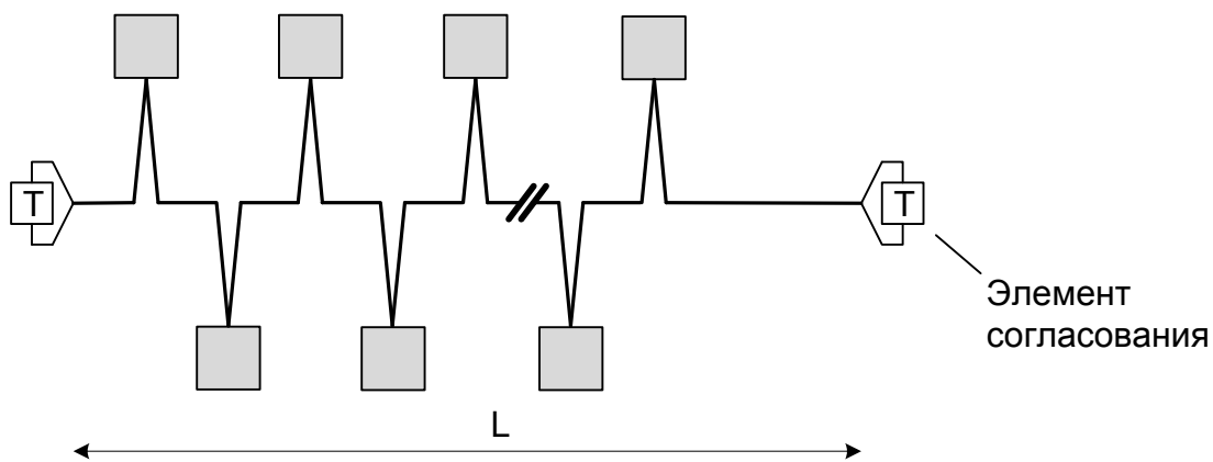
Рисунок 2 Шина без отводов
