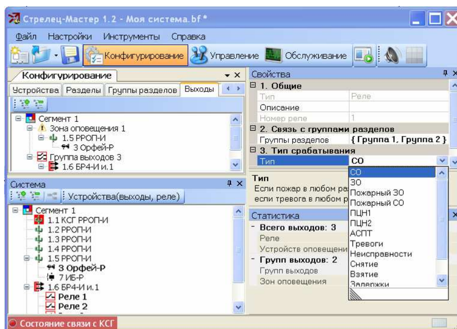
Рисунок 28 Конфигурирование событийных условий срабатывания выходов
