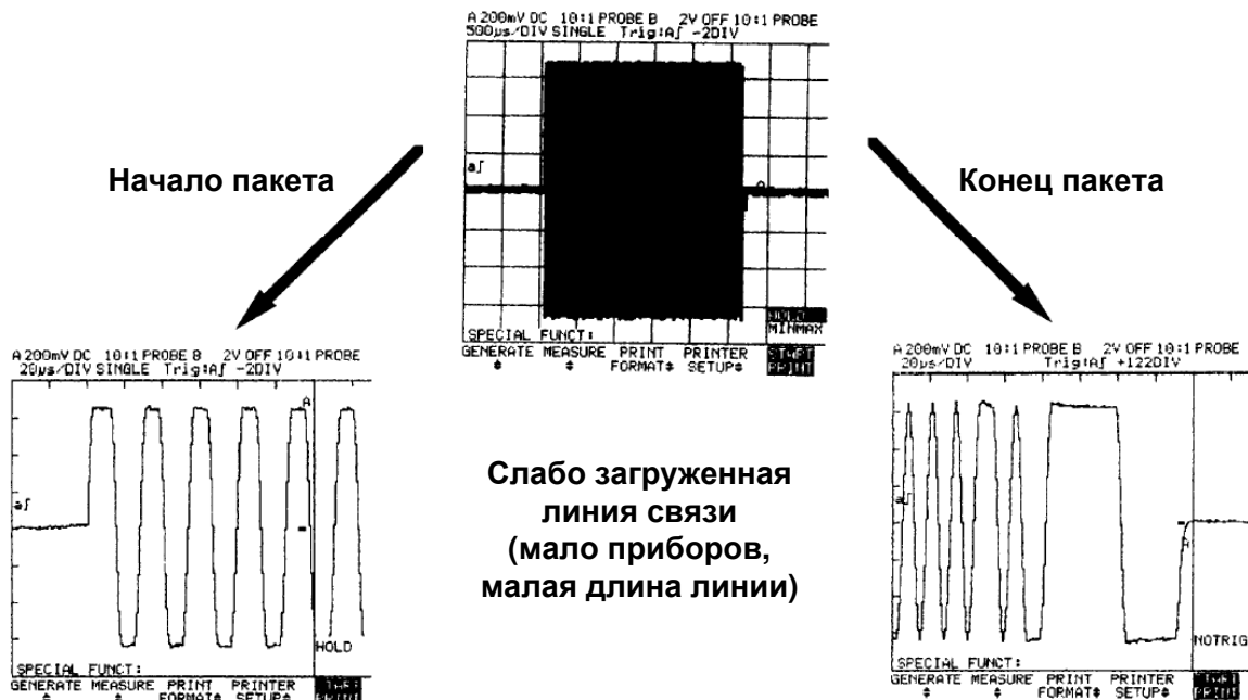
Рисунок 33 Типичная осциллограмма сигнала при слабой загрузке линии связи
