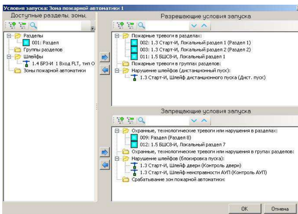
Рисунок 30 Условия запуска и запрета запуска зоны пожарной автоматики
