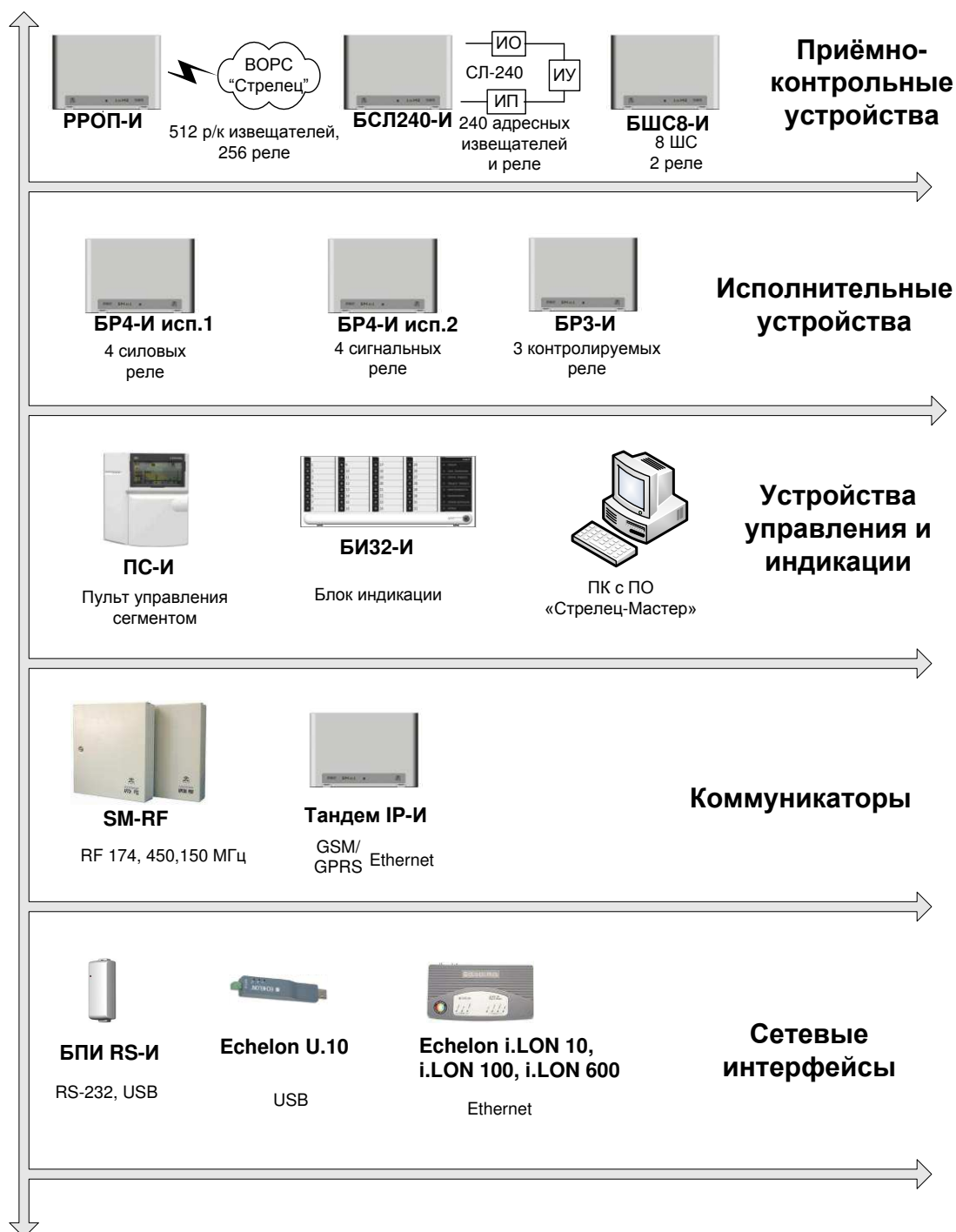
Рисунок 6 Состав оборудования сегмента
