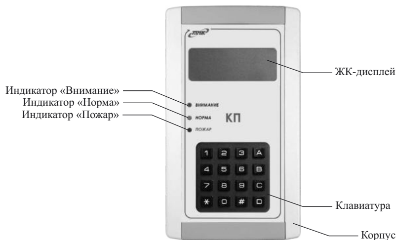
Рис. 6.12. Внешний вид КП-RS и КП-RF
