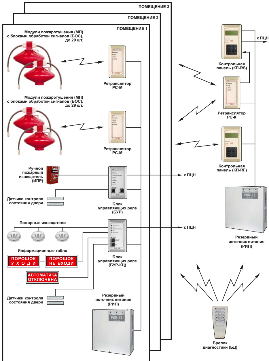
Рис. 4.4. Структурная схема АУП «Гарант-Р» ПО-2
