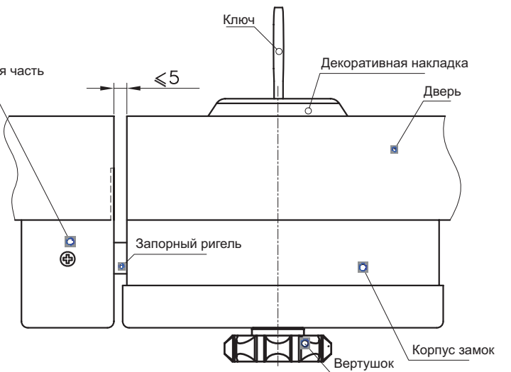
Схема расположения замка и его ответной части
