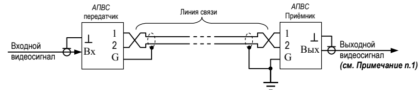
Рис.3 Схема включения АПВС-5М при невозможности заземления на передающей стороне
