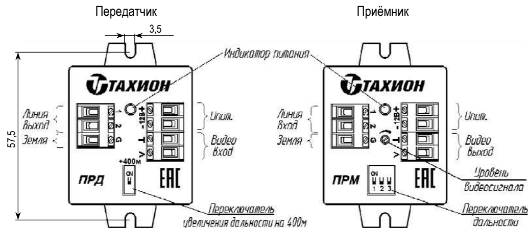
Рис.1 Устройство АПВС-5М
