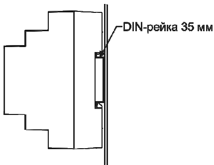
Рисунок 2 – Установка изделия
