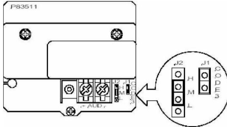
Рис 3: Расположение переключателей для выбора необходимого режима работы оповещателя.
